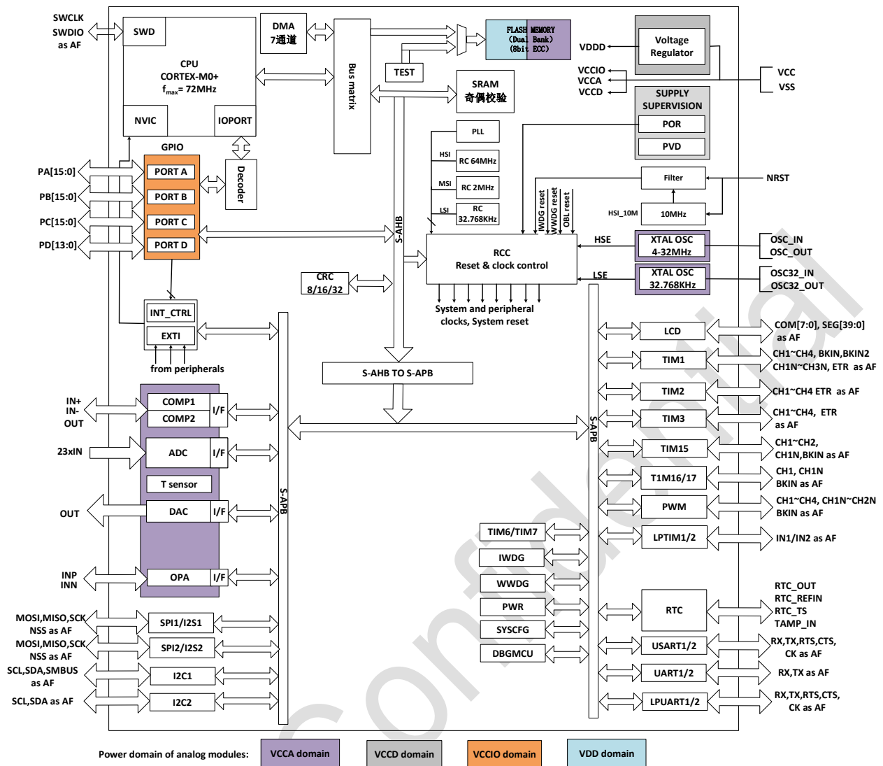
图 1-1 功能模块
