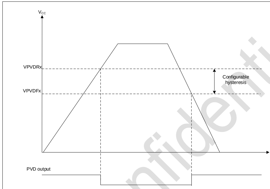
图 2-3 PVD 阈值
